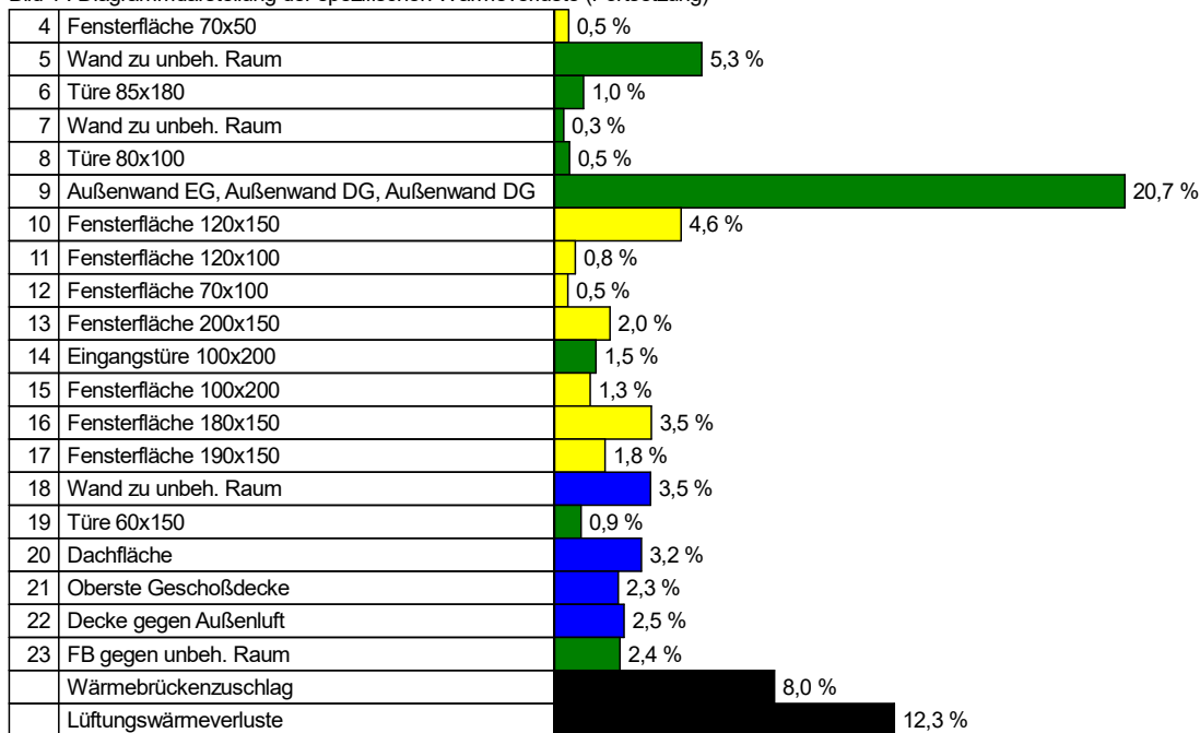
Bild 1 : Diagrammdarstellung der spezifischen Wärmeverluste (Fortsetzung)
